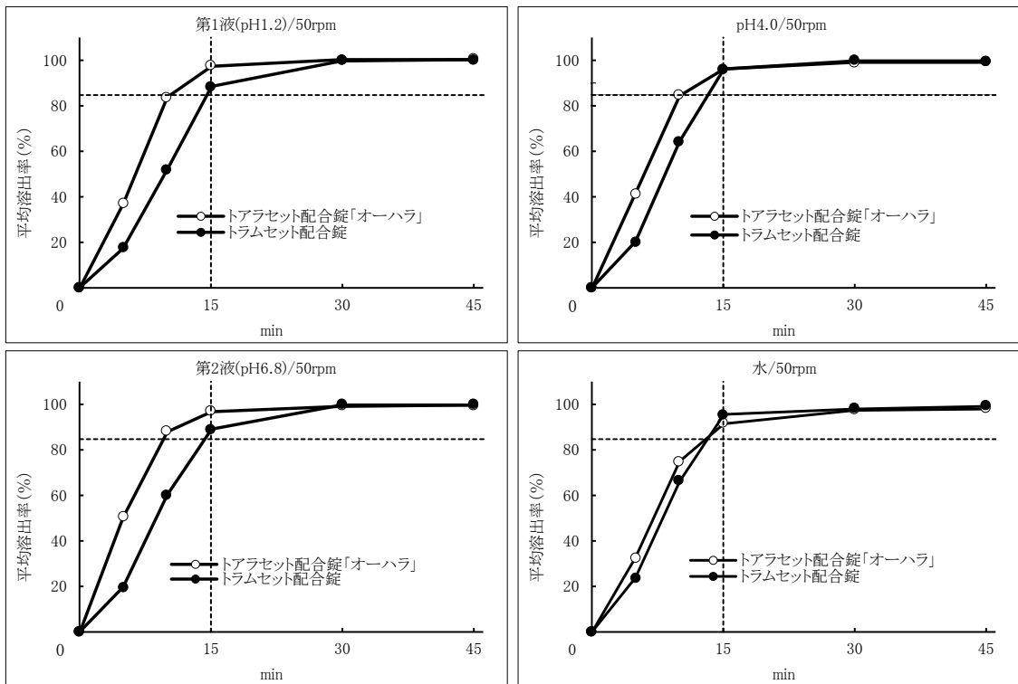
(溶出曲線)
