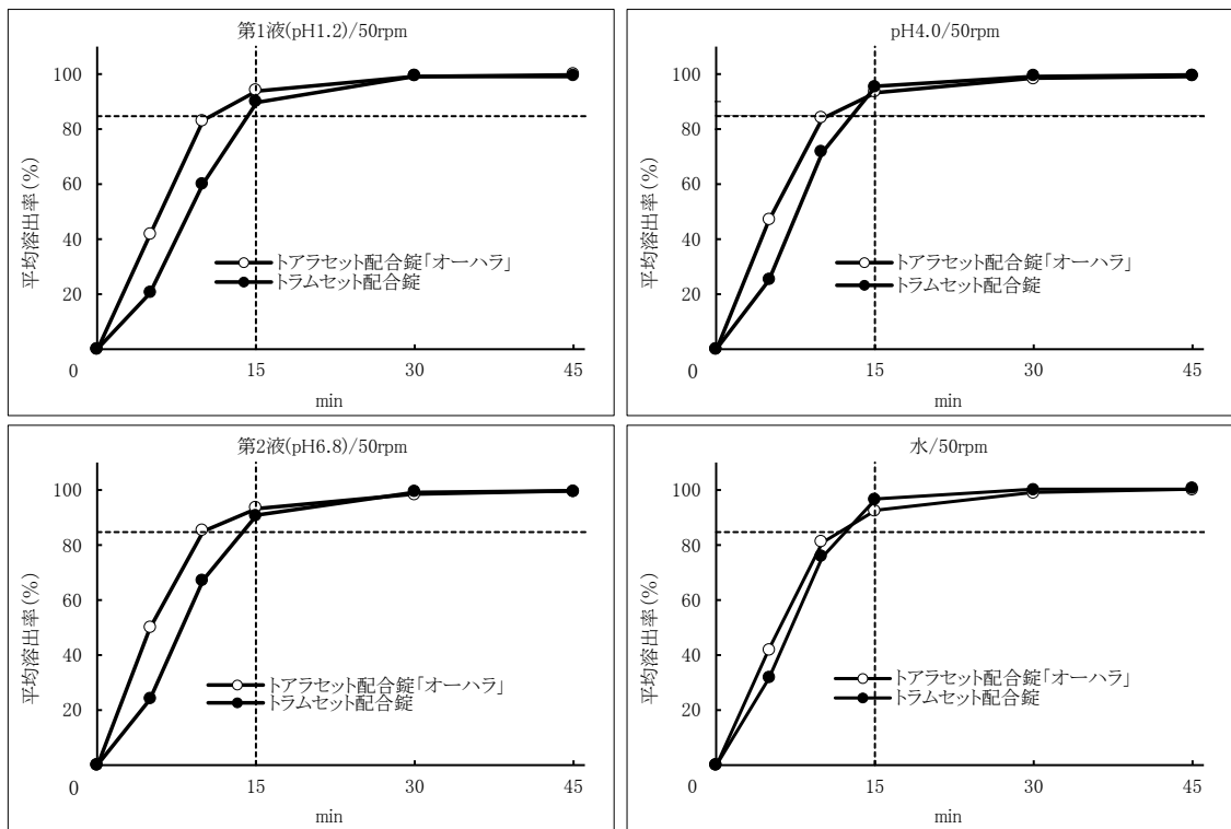
(溶出曲線)
